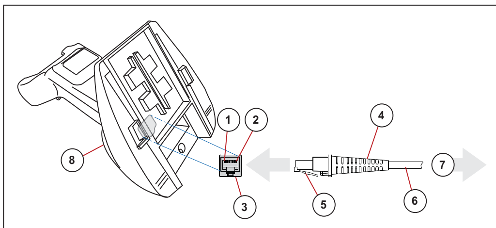
Рис 15. Стандартные разводки выводов кабелей: базовая станция
